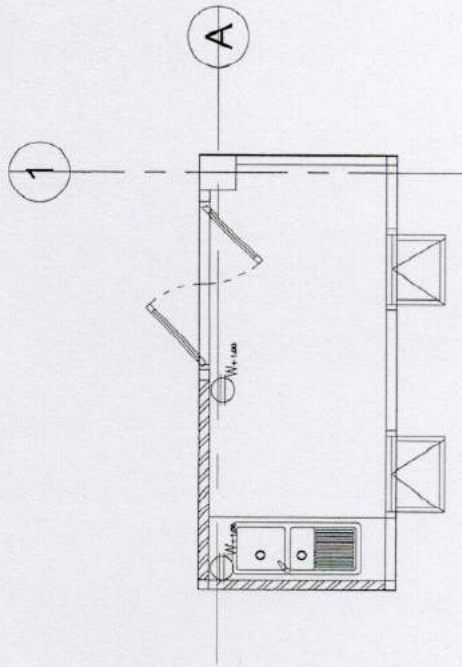
แปลนไฟฟ้าและสื่อสาร SCALE 1:50
