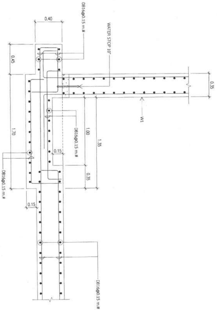
แบบขยายการเสริมเหล็กของ SUMP 1:25
